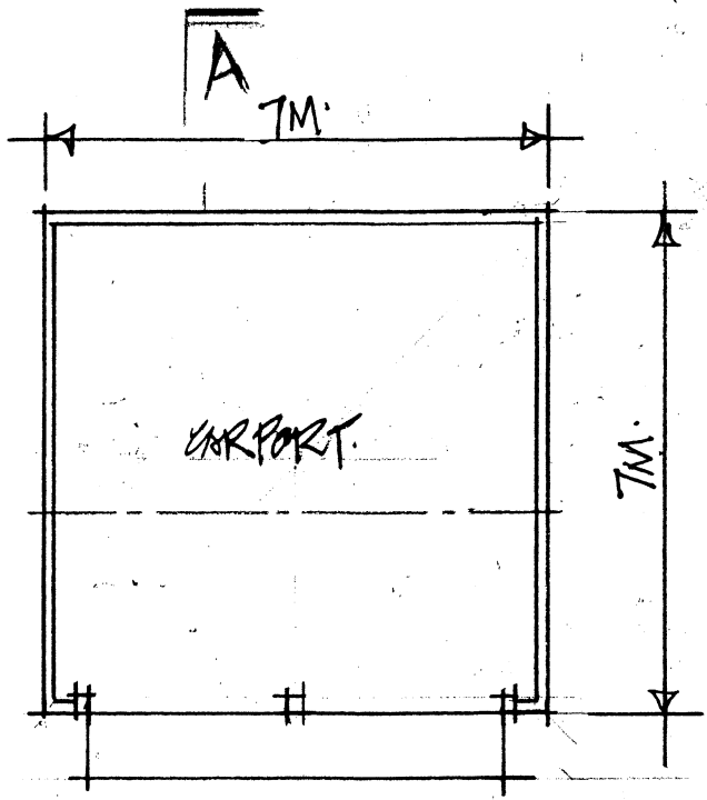
PLAN 1:100
