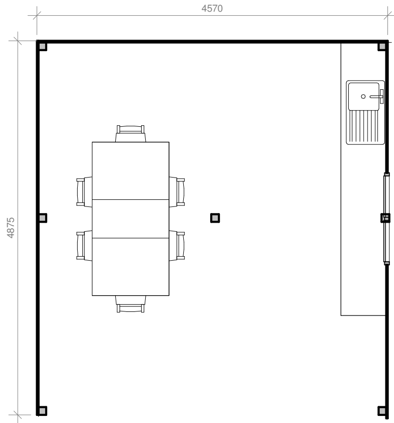
Floor Plan 1 : 50
