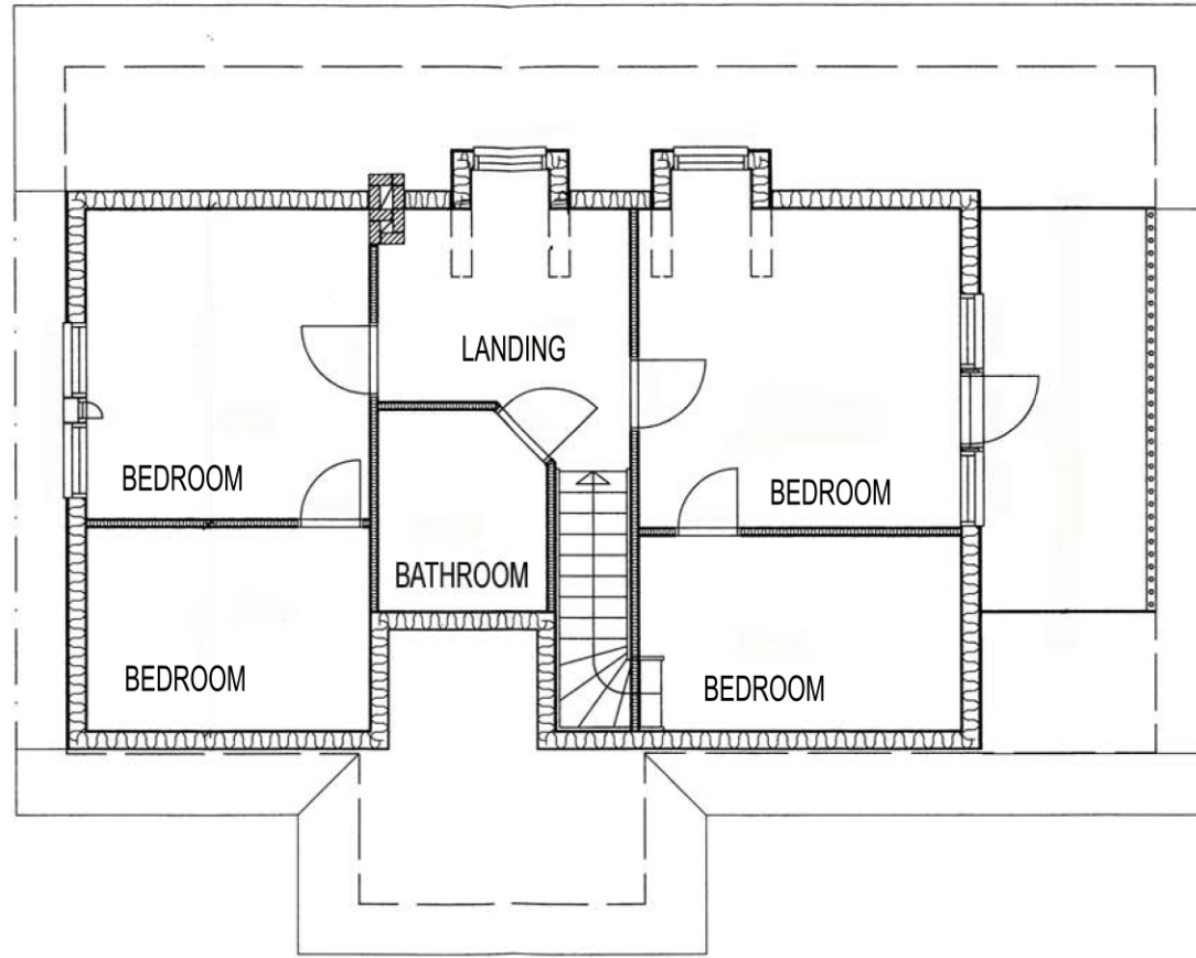
F.F. PLAN
