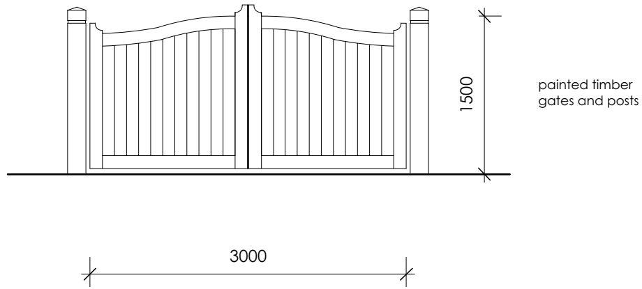
ELEVATION 1:50
