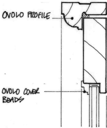
door details 1:5 SOLID EUROPEAN OAK
