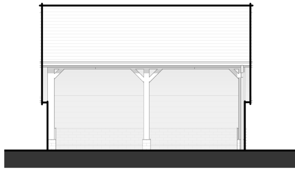
front 1 : 100
