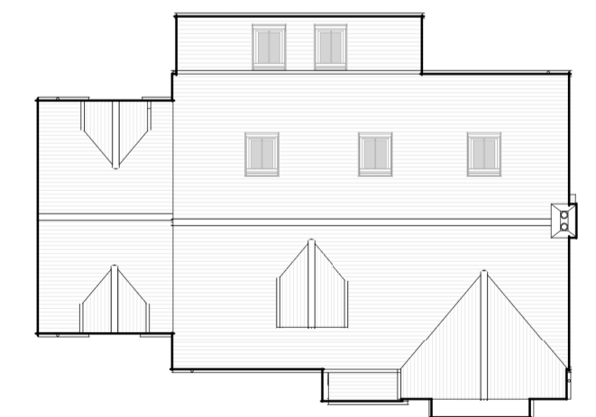
roof plan 1 : 200
