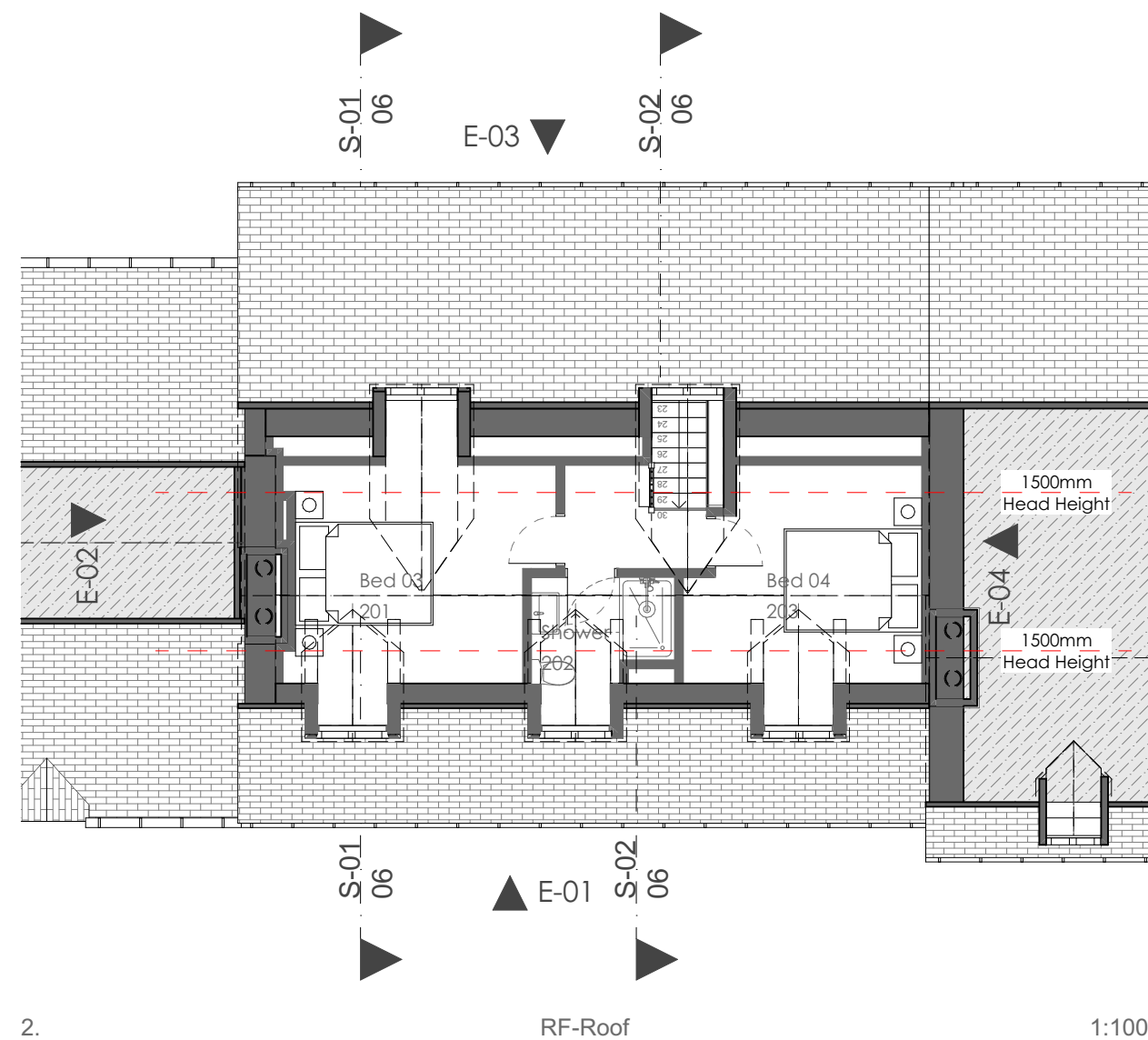
2. RF-Roof 1:100
