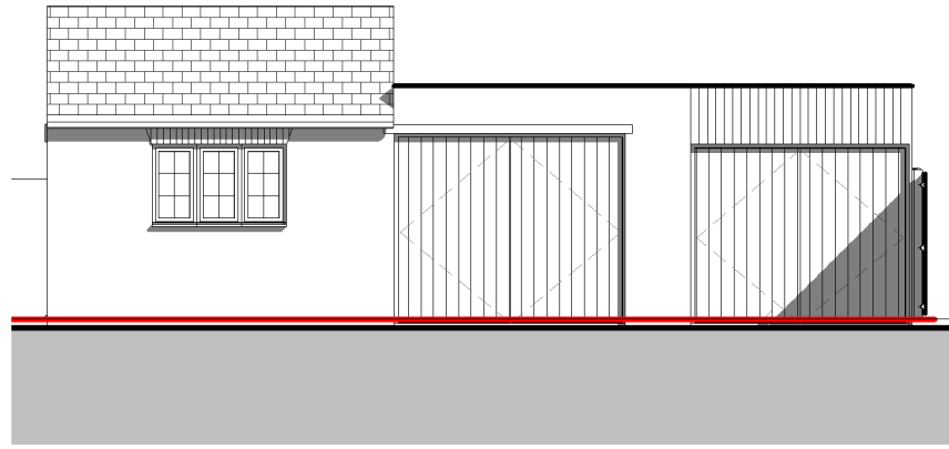
2 North 1 : 100
