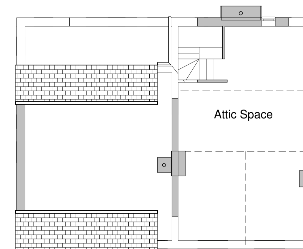
9 30 Eaves Level 1 : 100
