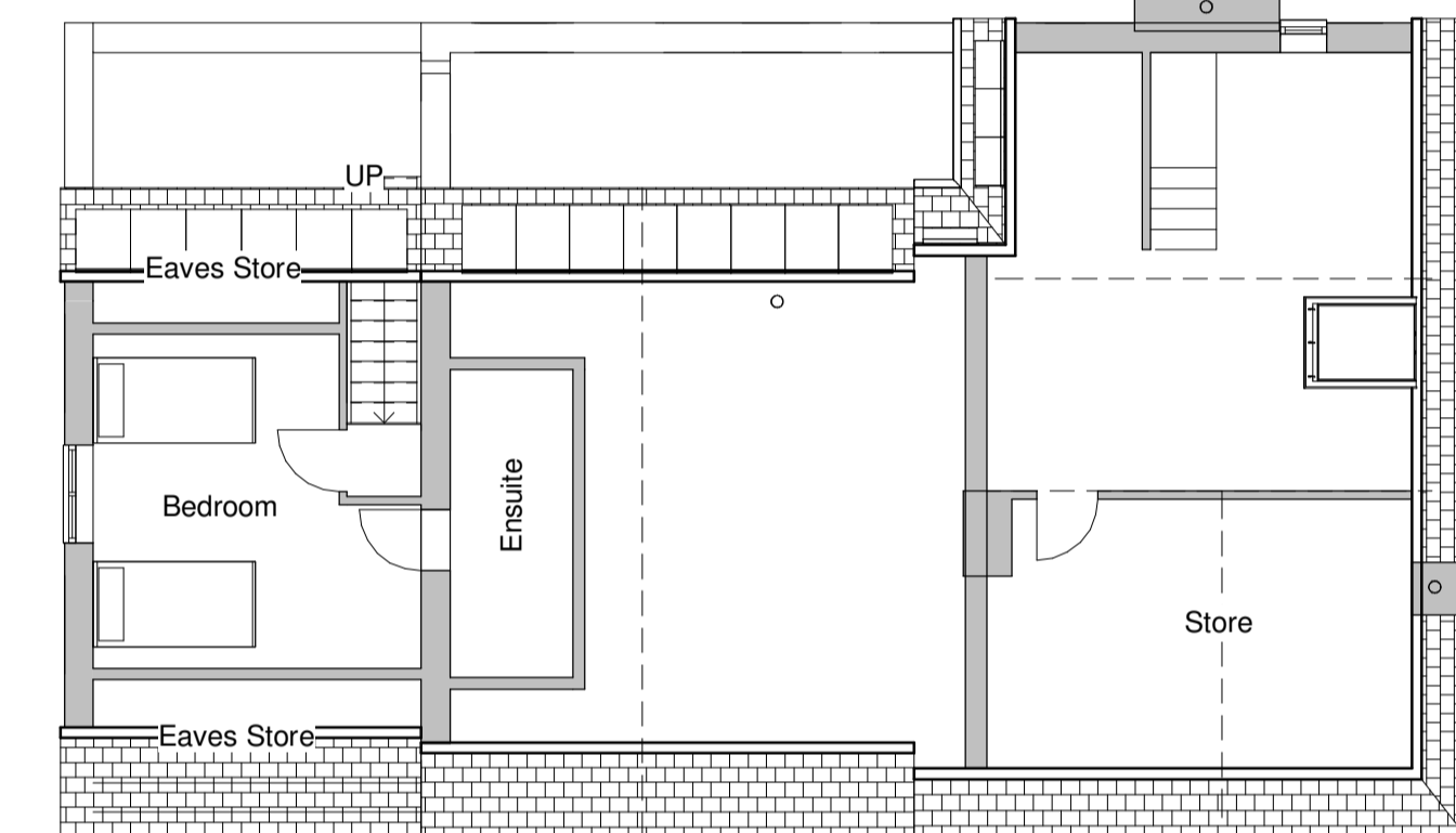
9 30 Eaves Level 1 : 100
