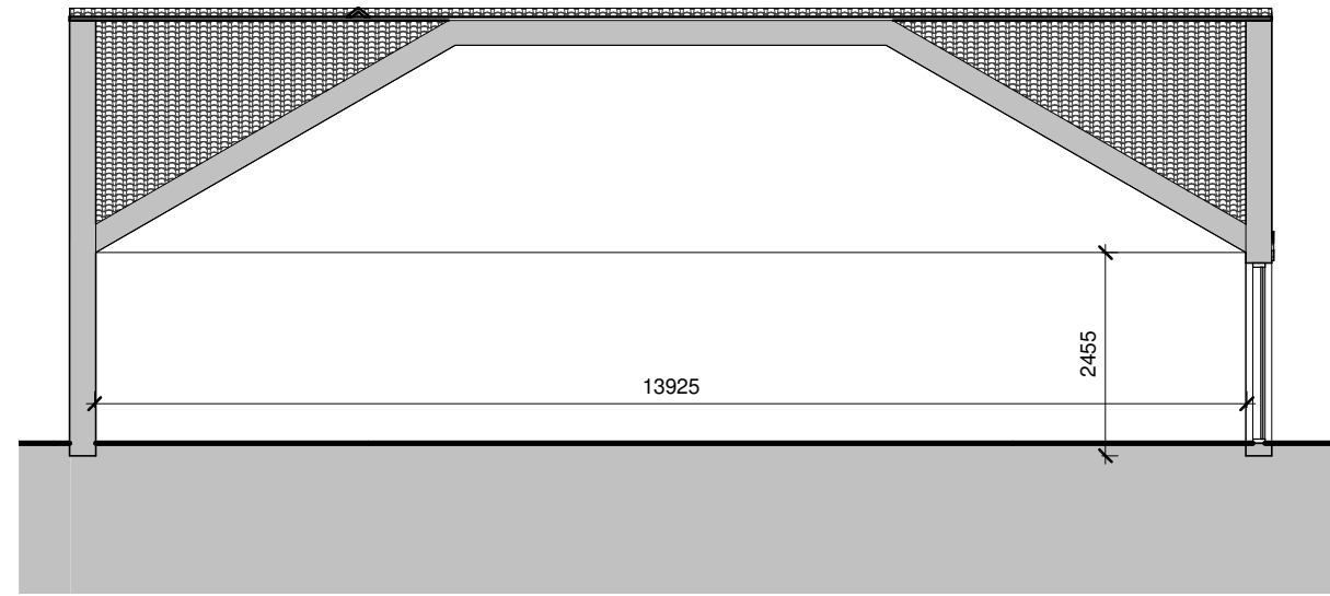
1 Section 1 PP-12 1 : 100
