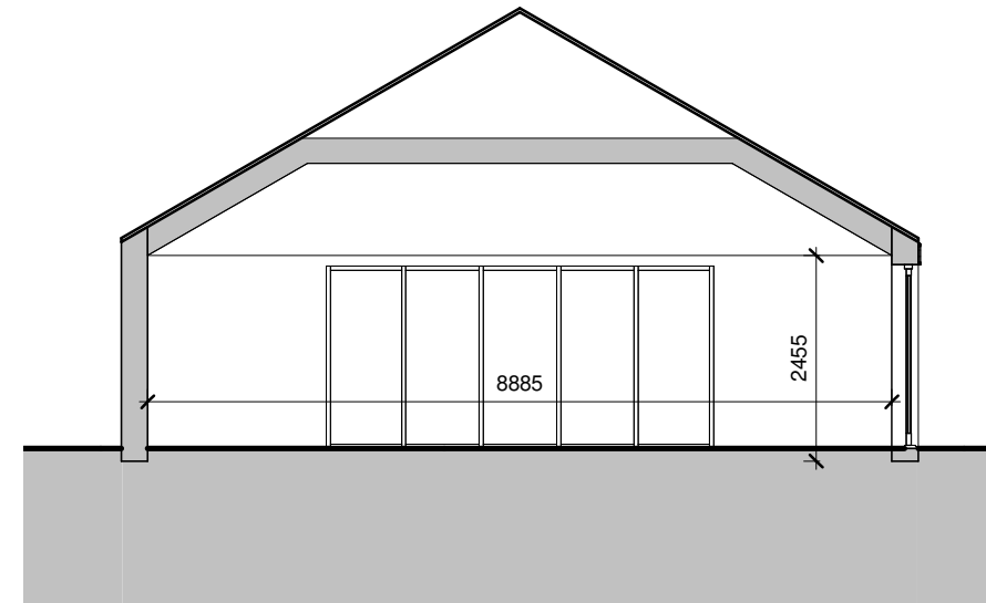
2 Section 2 PP-12 1 : 100
