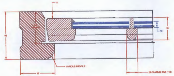
JAMB DETAIL
