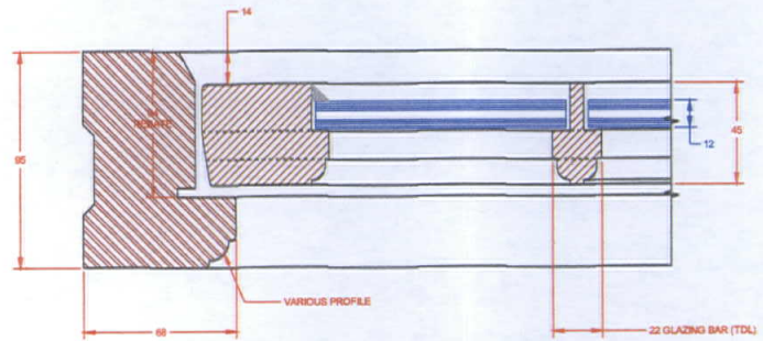
JAMB DETAIL
