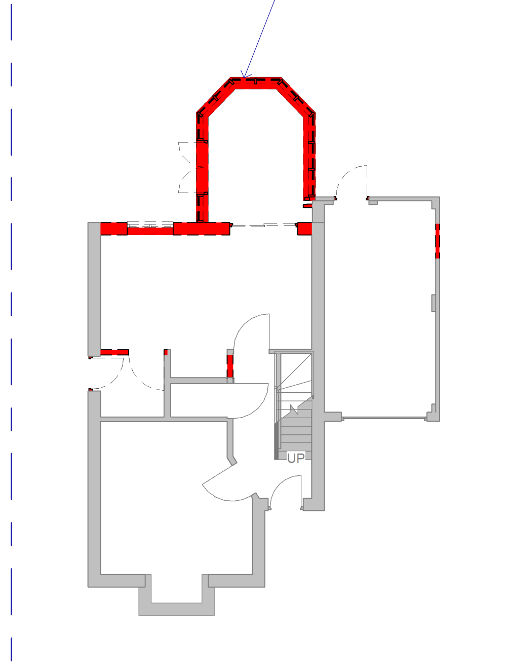
1 Demolition Plan 1 : 100
