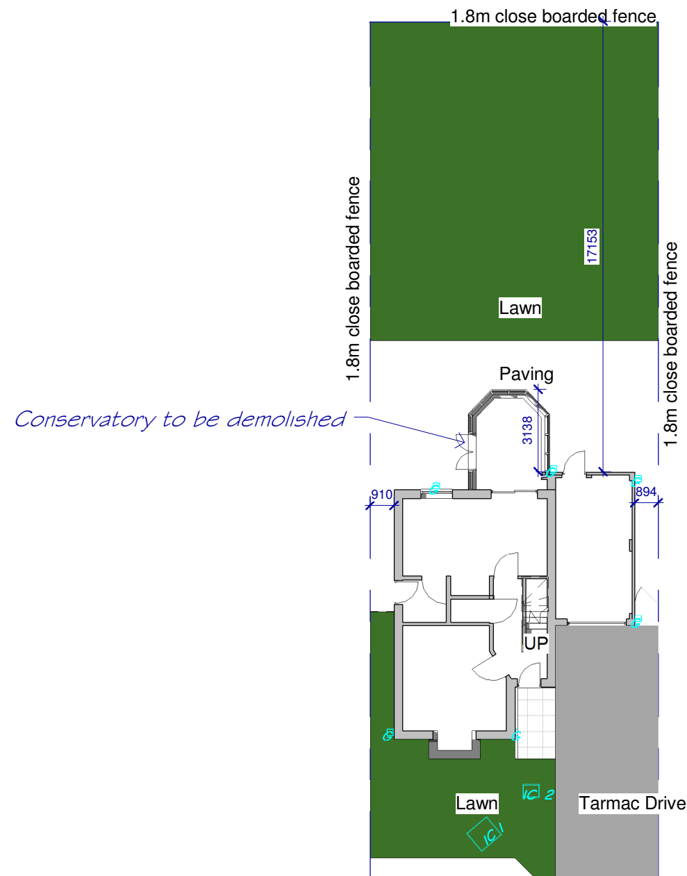
1 Existing Site Layout 1 : 200
