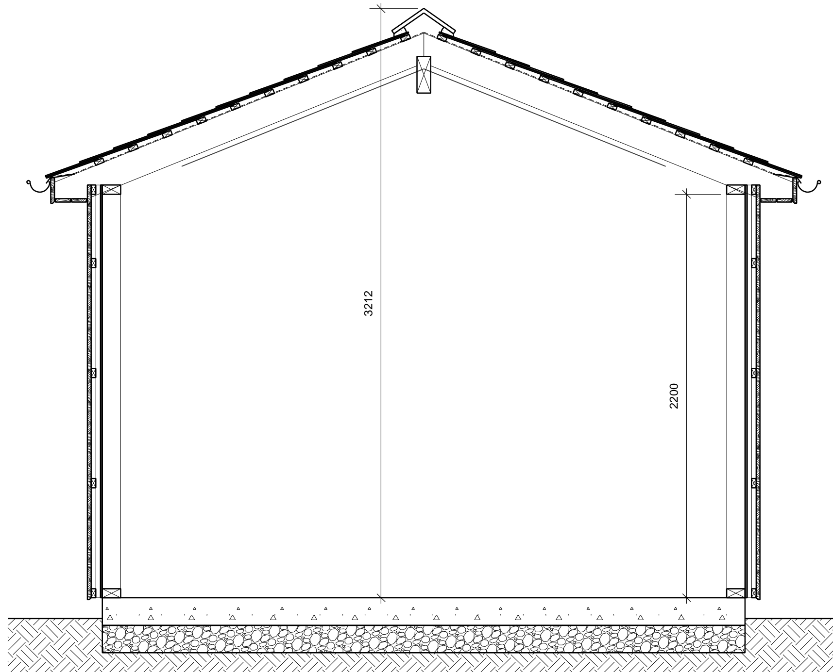
Section A-A
