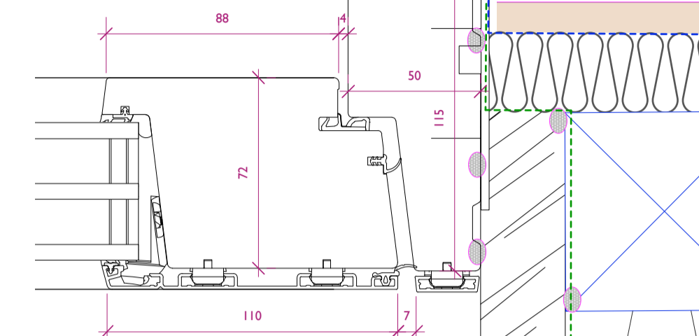
JAMB
