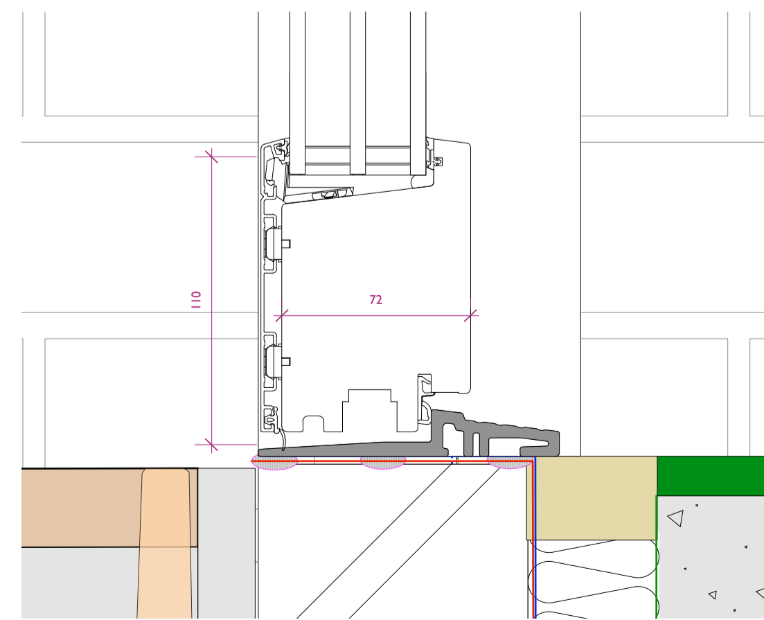
DOOR SECTION DETAILS 1:2 Scale
