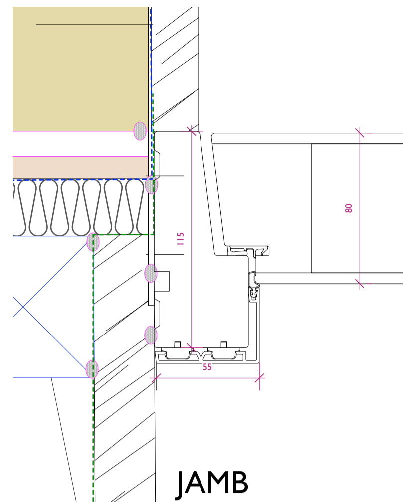
PLAN DETAILS 1:2 Scale SOLID DOOR
