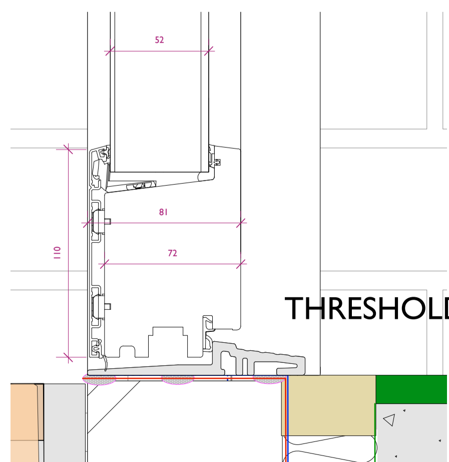
DOOR SECTION DETAILS 1:2 Scale
