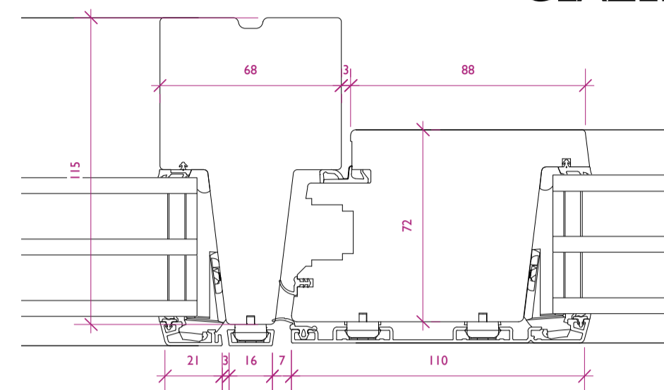
SIDELIGHT
