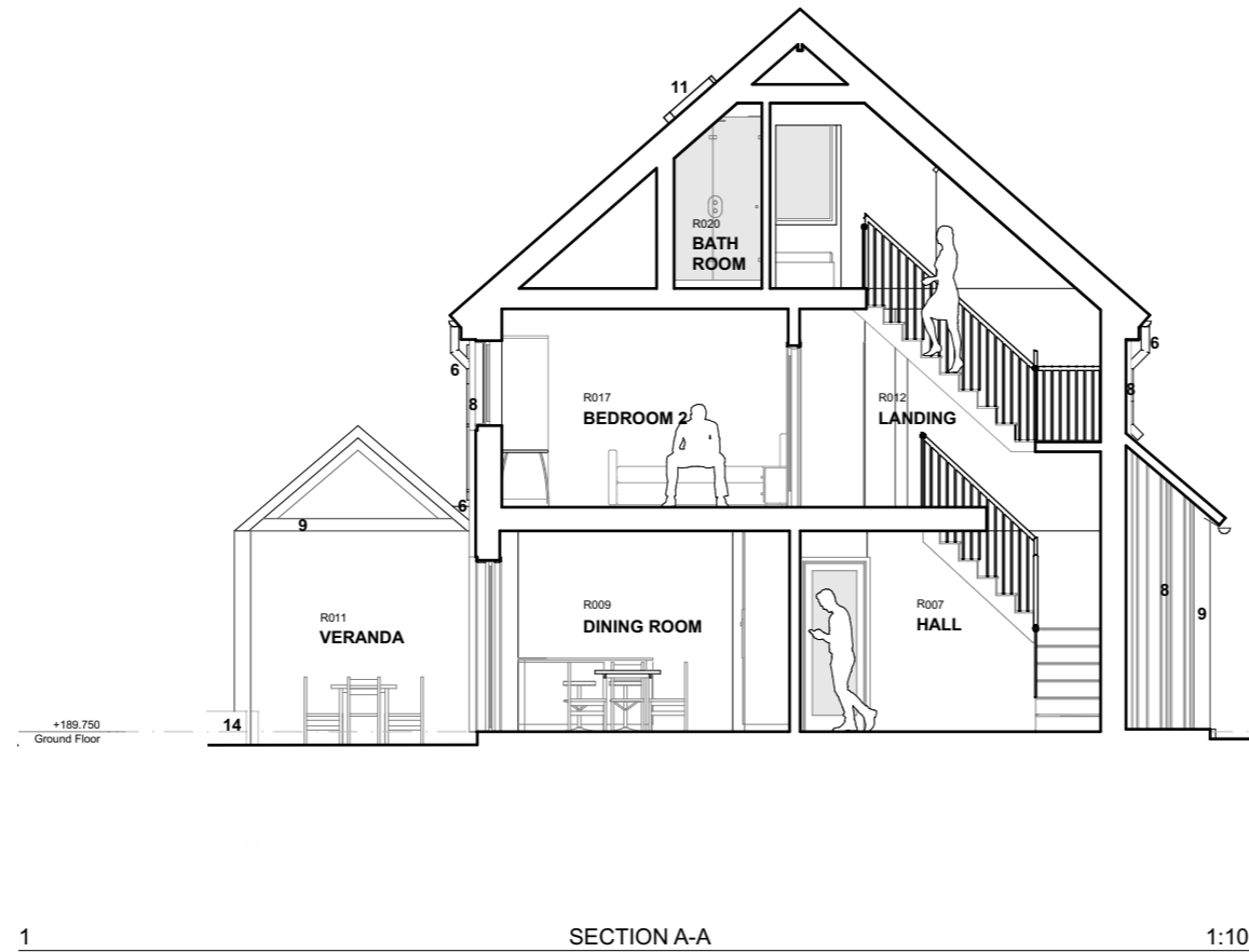
1 SECTION A-A 1:100
