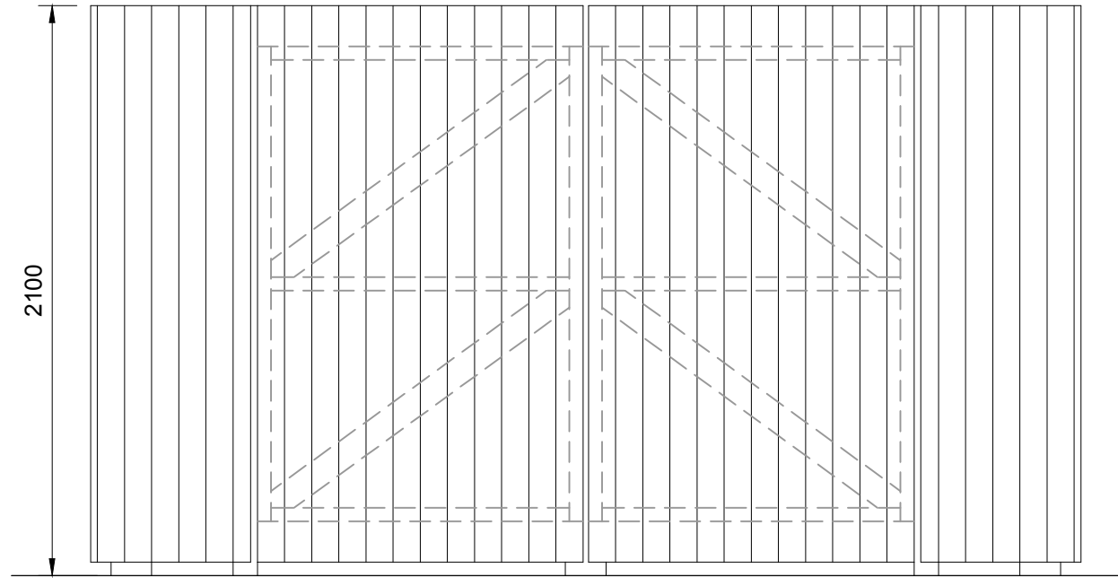
ELEVATION
