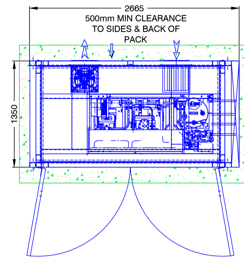
SCM-FRIGO DT CO2 LOW NOISE PACK SCALE 1:30
