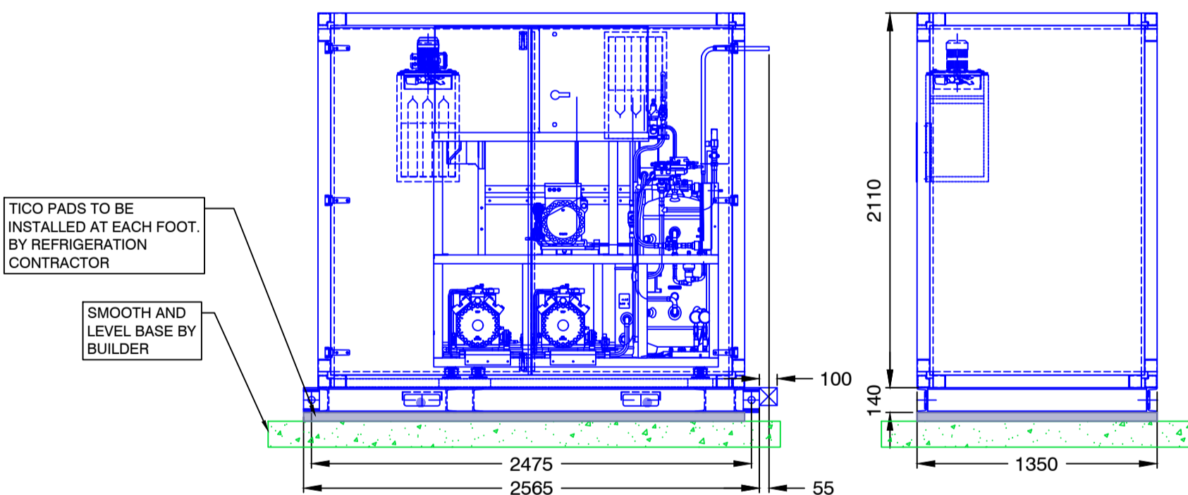
SCM-FRIGO DT CO2 LOW NOISE PACK SCALE 1:30
