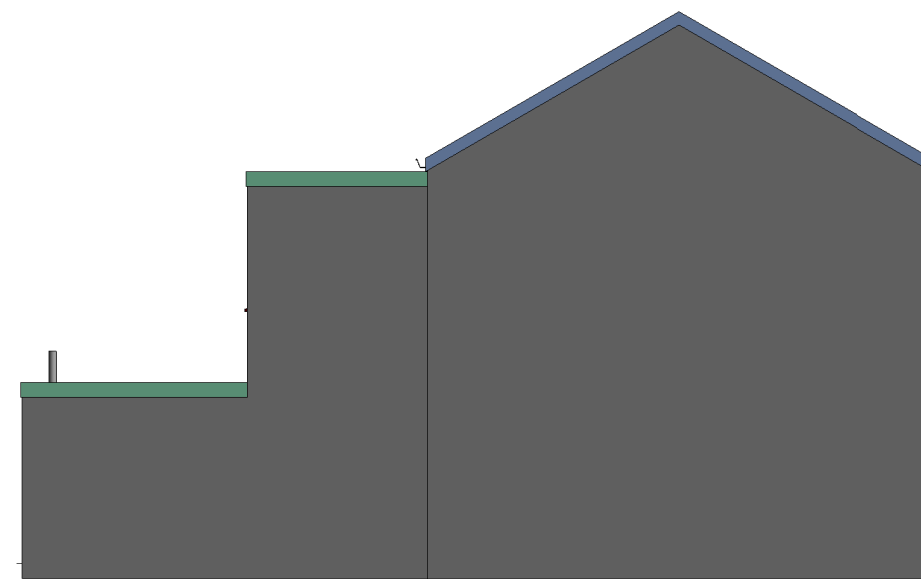
2 SW elevation 1 : 100
