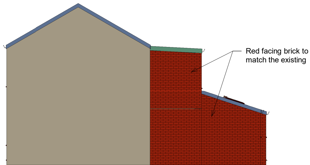
1 NE elevation 1 : 100
