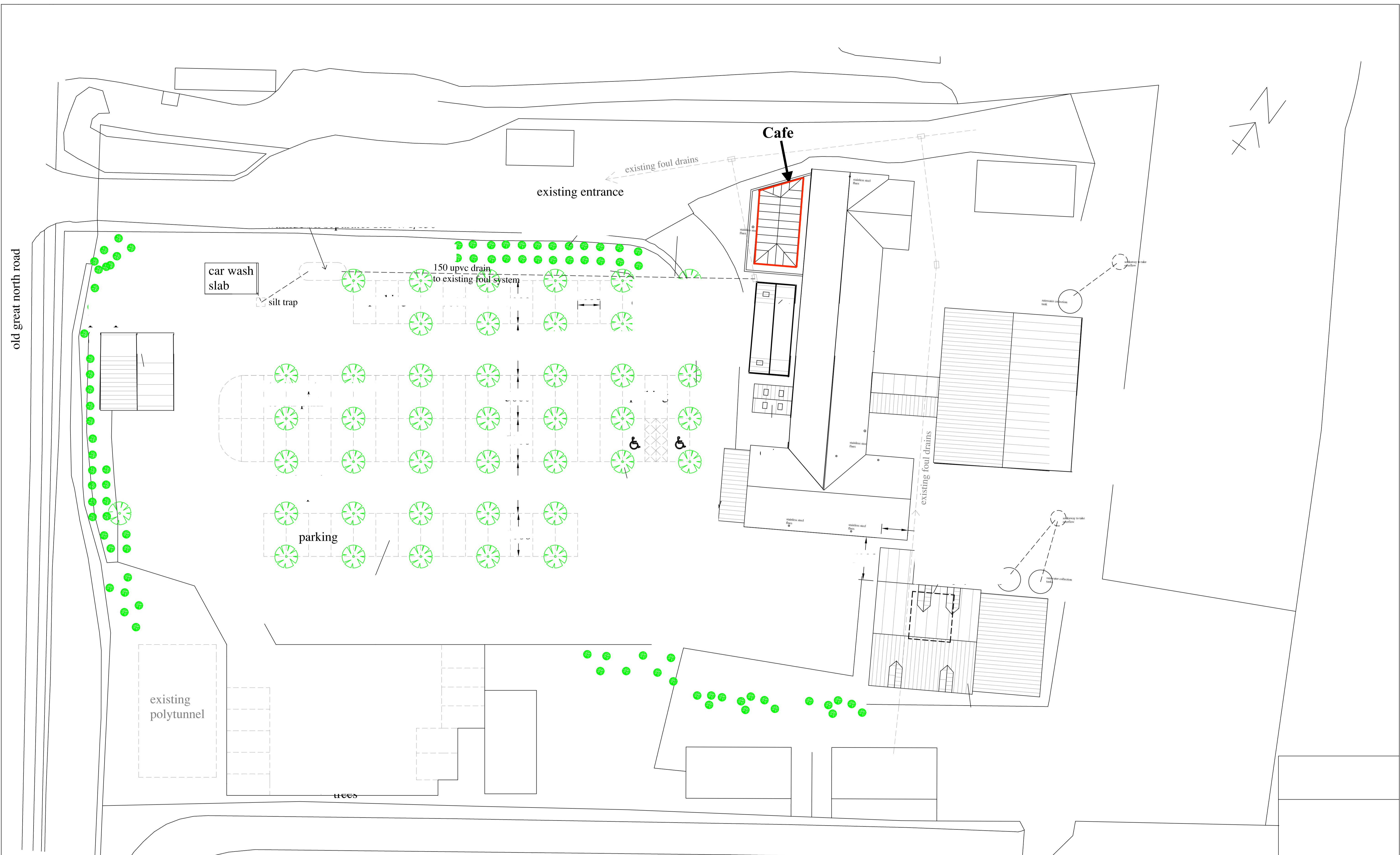
SITE PLAN 1 : 200
