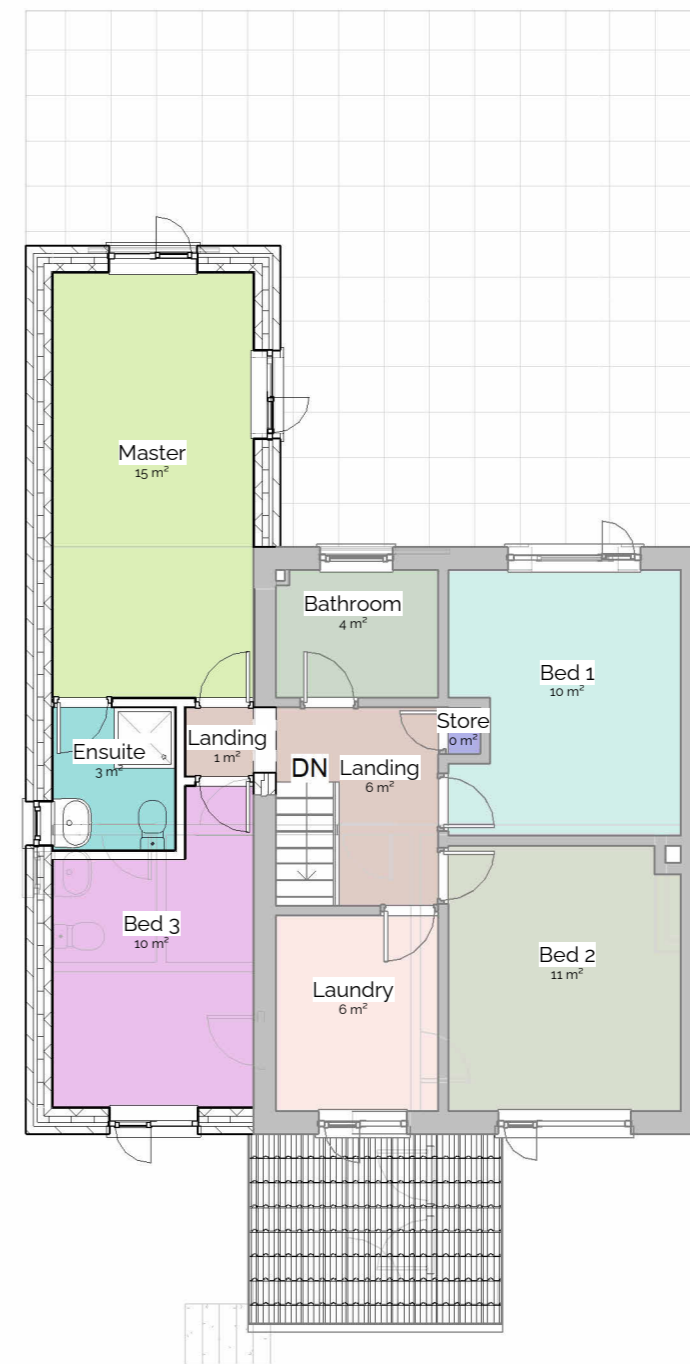
2 First 1 : 100
