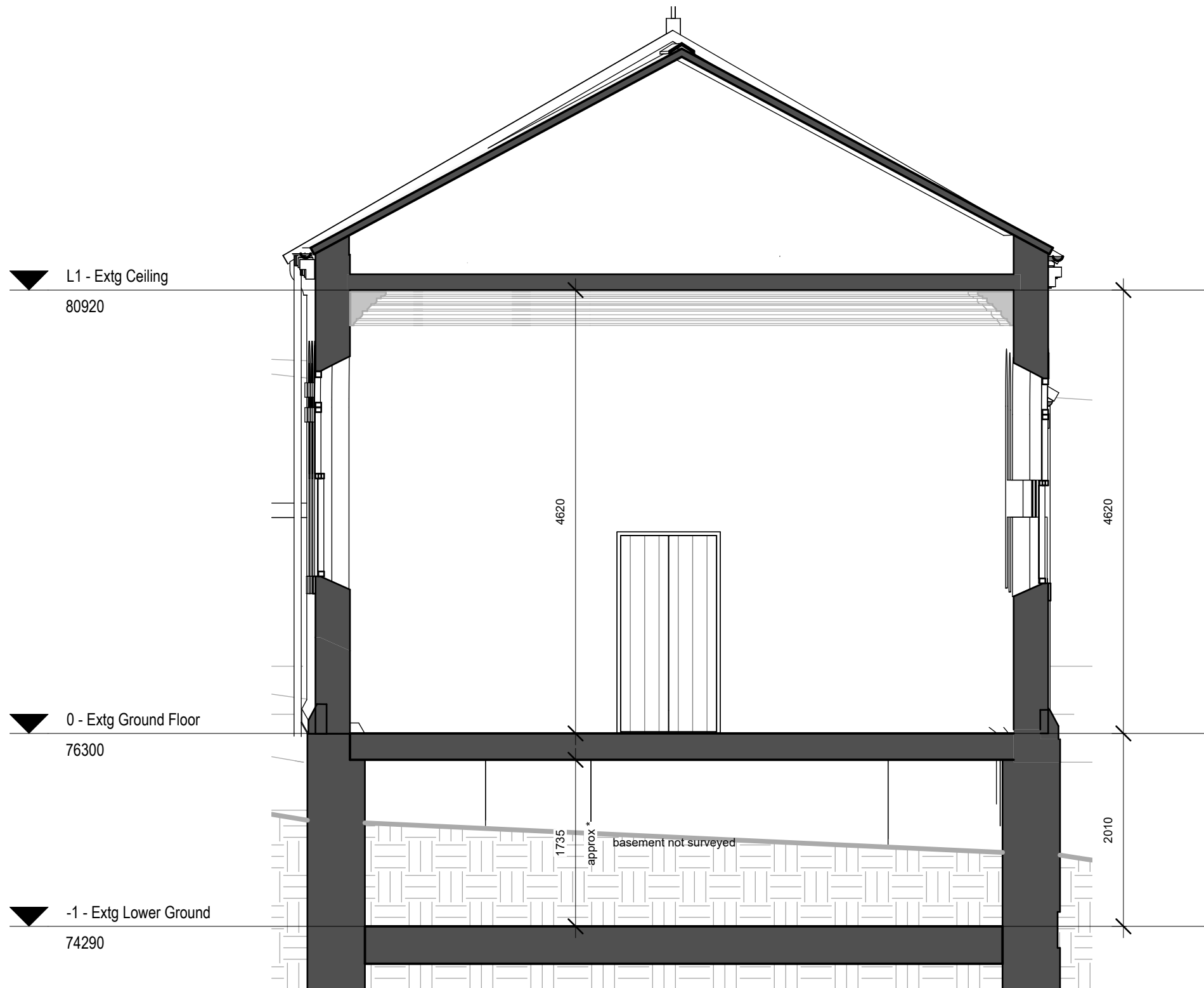
1 Existing Section 1 : 50
