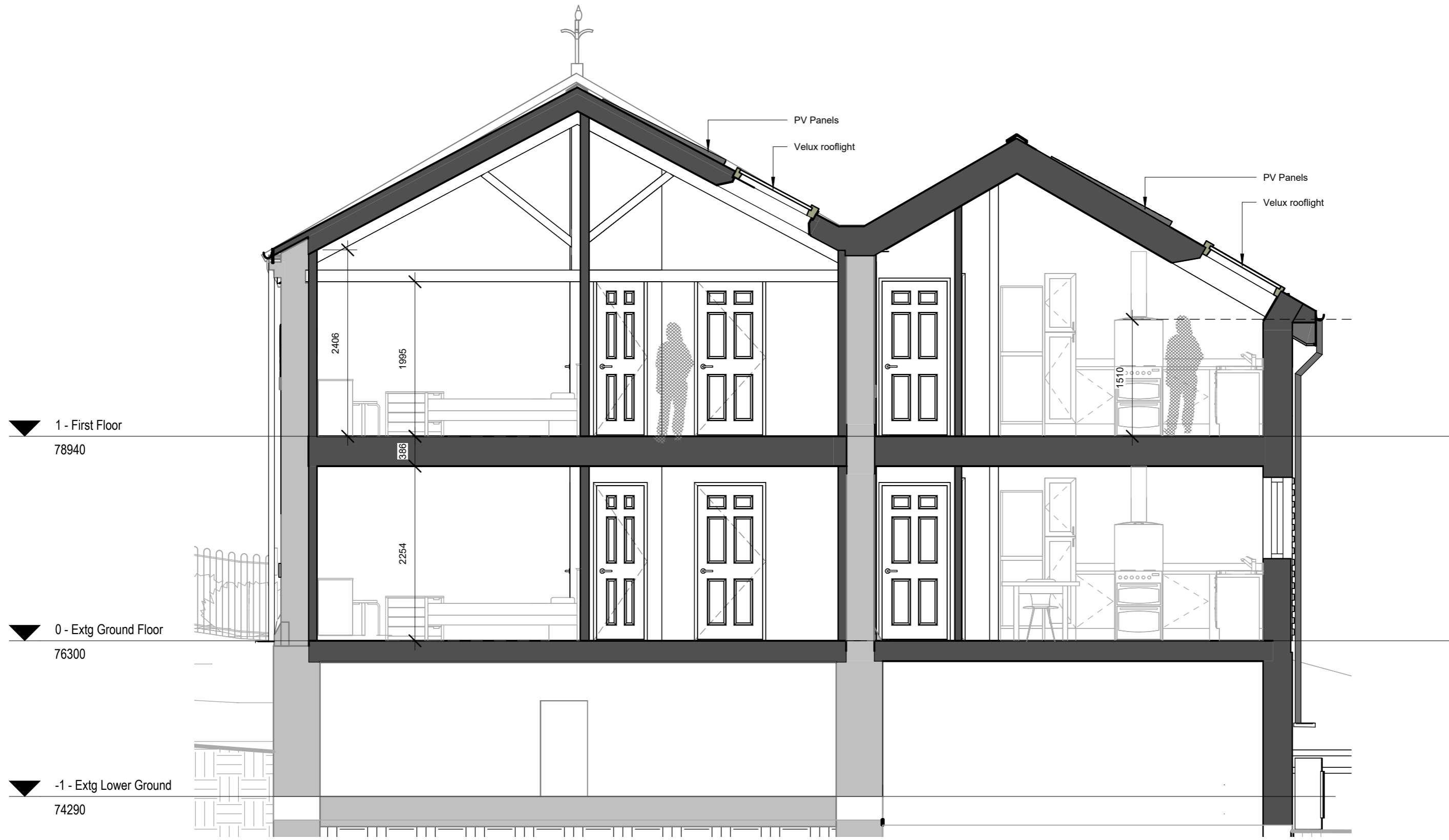
1 Section 2 1 : 50
