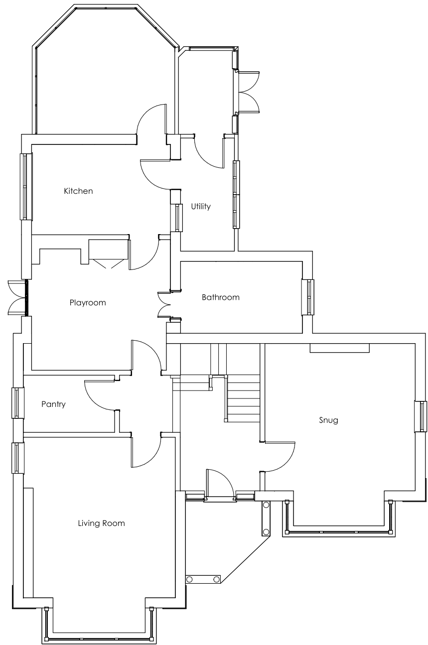
1 LO FFL 1 : 50
