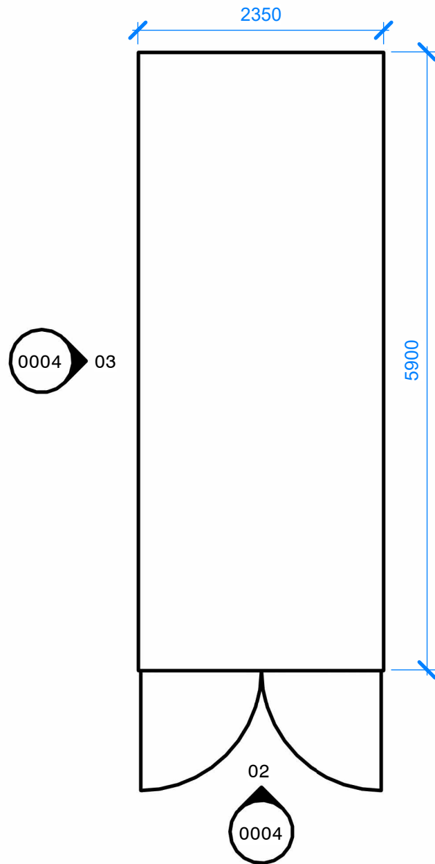
1 Container Plan 1 : 50
