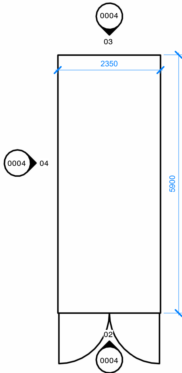
1 Container Plan 1 : 50
