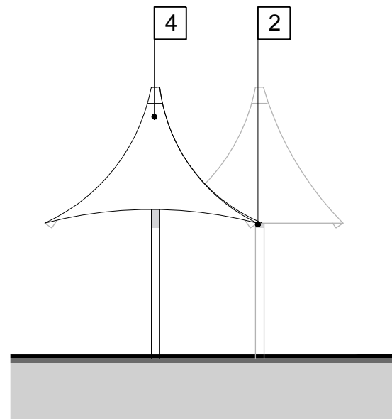
Elevation B-B
