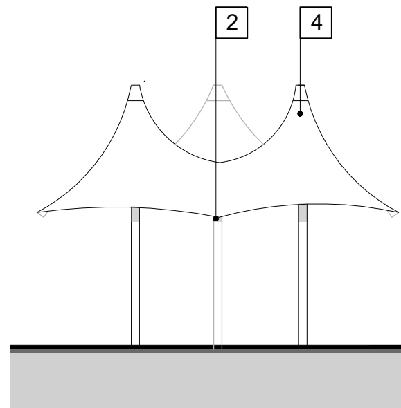
Elevation C-C
