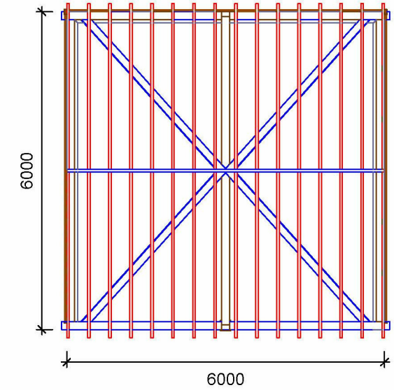
Scale: 1 : 100 PLAN_ELEVATION
