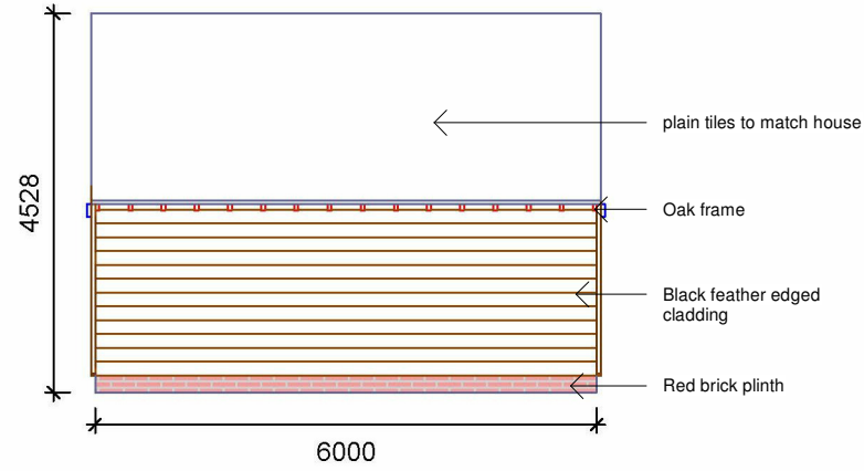
Scale: 1 : 100 REAR_ELEVATION
