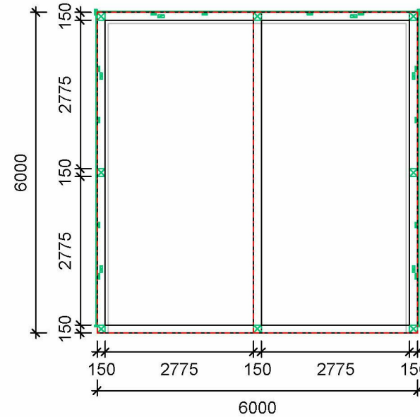
Scale: 1 : 100 POST_ELEVATION
