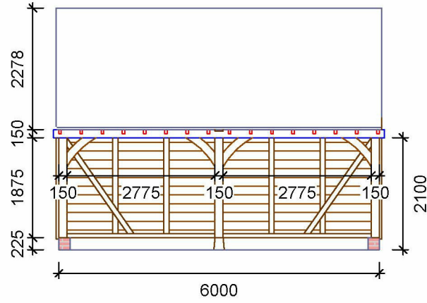
Scale: 1 : 100 FRONT_ELEVATION
