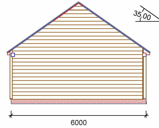
Scale: 1 : 100 LEFT_ELEVATION
