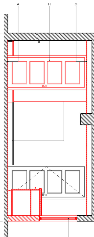
IRL - Existing - Elevation C 1:50
