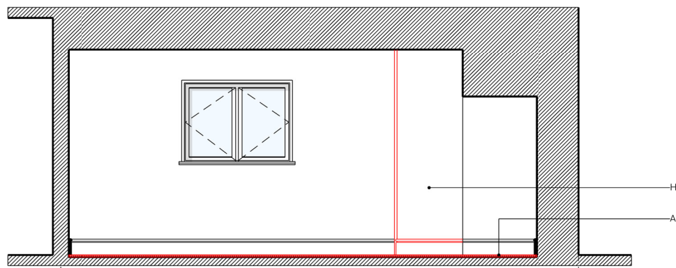
IRL - Existing - Elevation A 1:50
