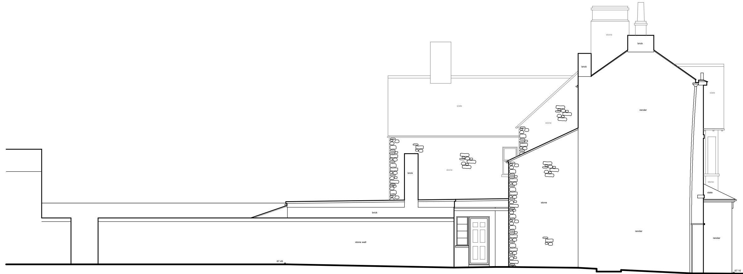
1 Existing west elevation Scale: 1:100
