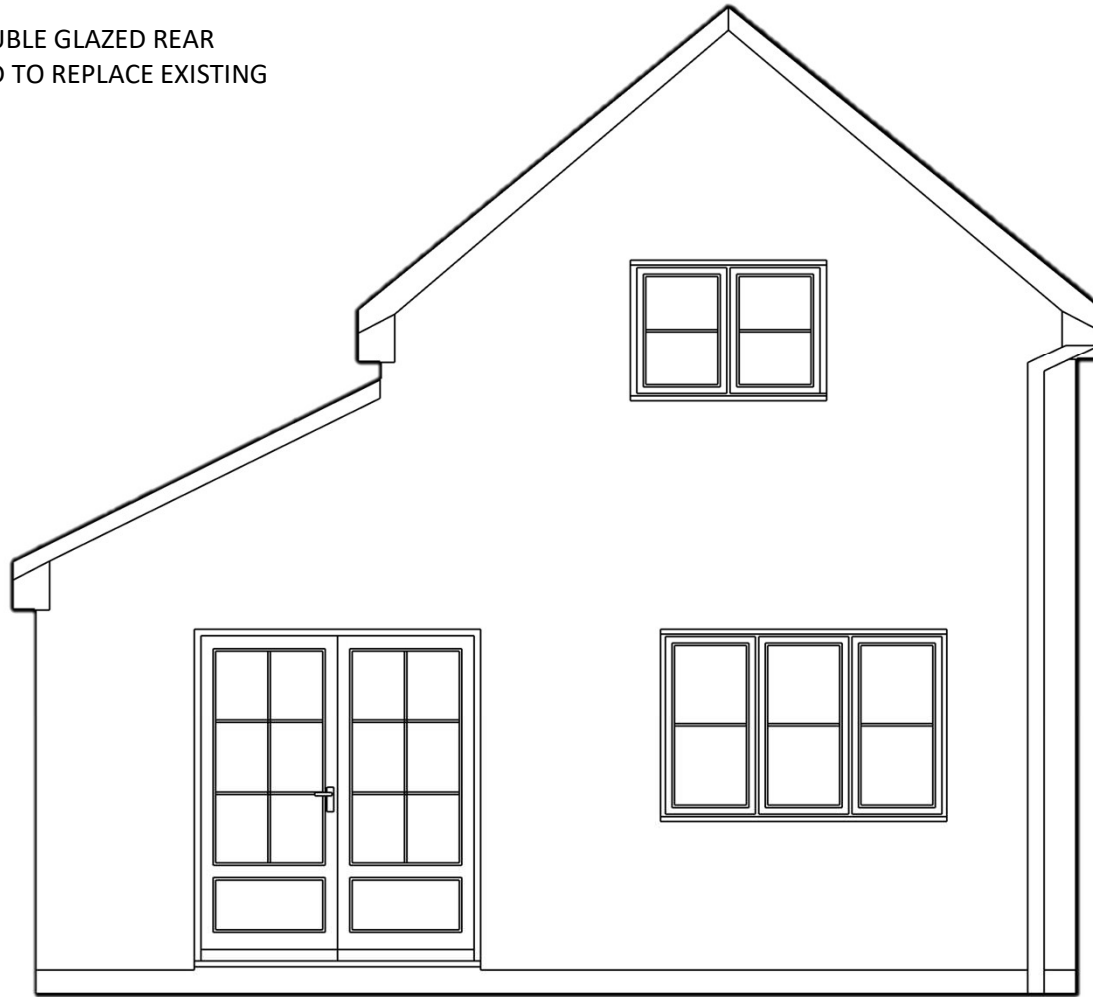
ELEVATION D-D
