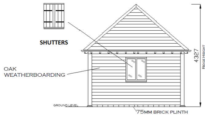
REAR ELEVATION N.E.
