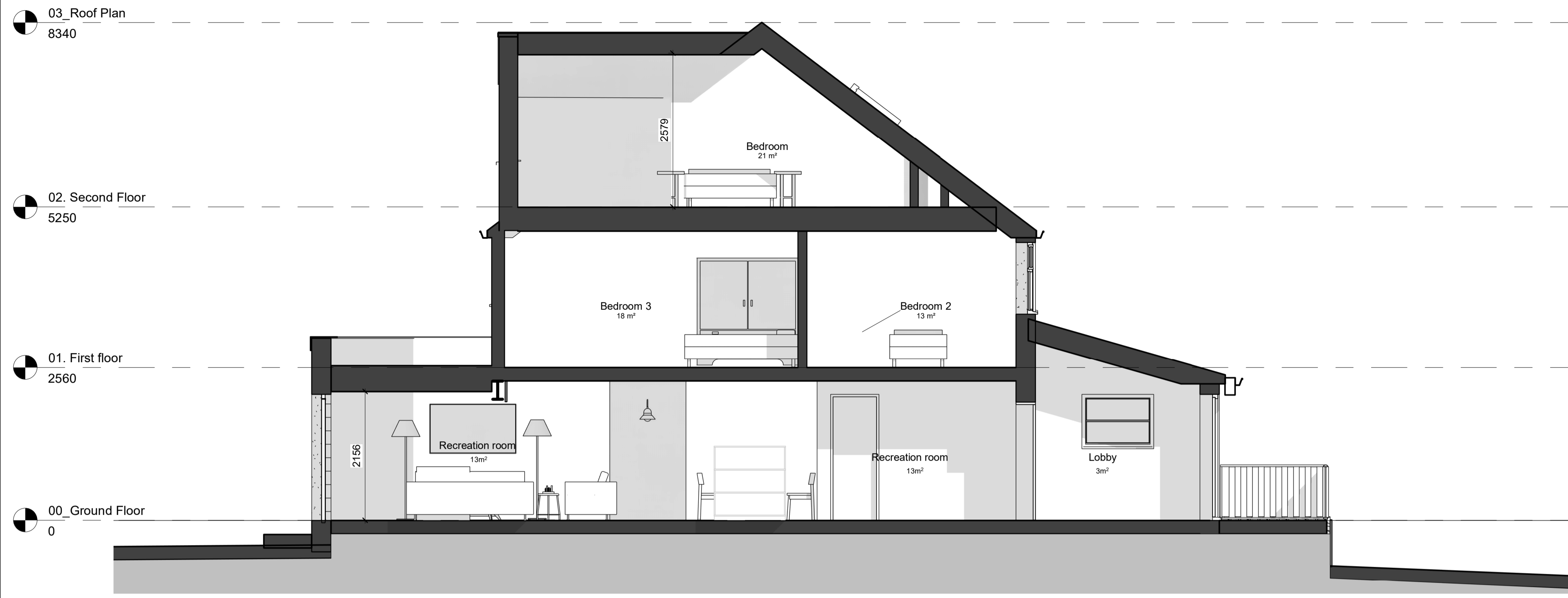
Section AA 1 : 50 @A1 1:100 @A3
