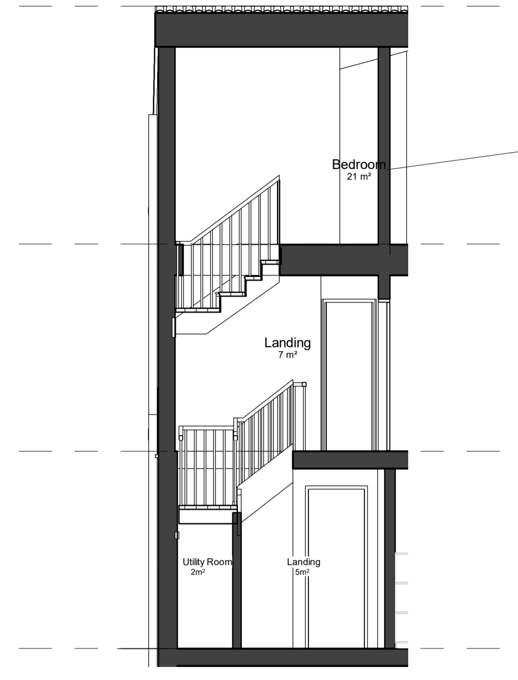
Section CC 1 : 50 @A1 1:100 @A3
