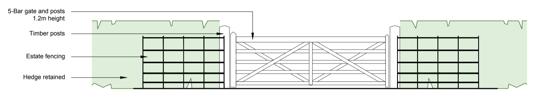
Gate Elevation Scale: 1:50
