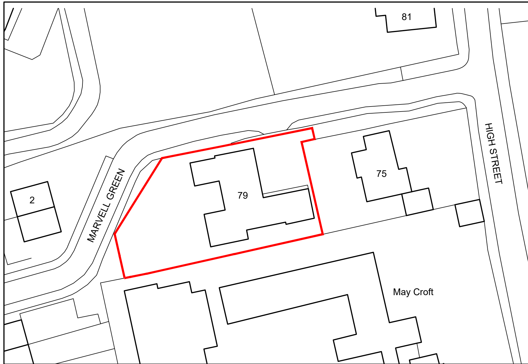
site plan - 1:500
