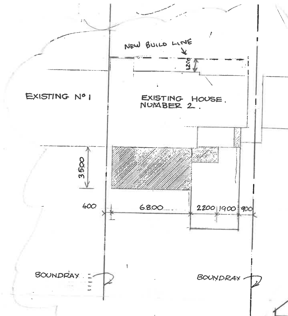
1:200 SITE PLAN.
