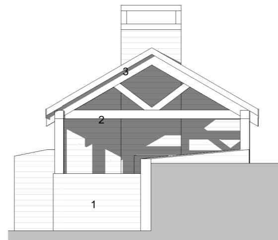
East 1 : 100
