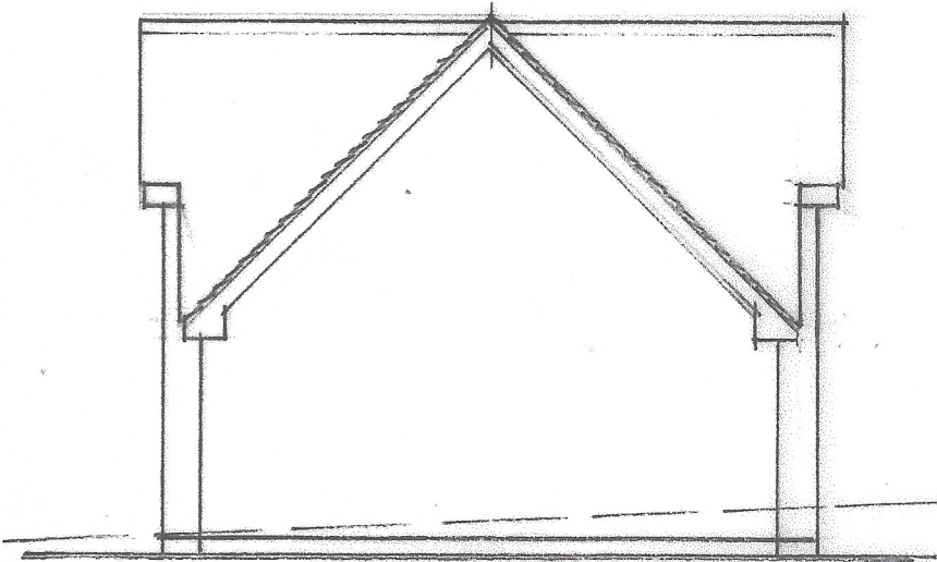
LH SIDE 1:100
