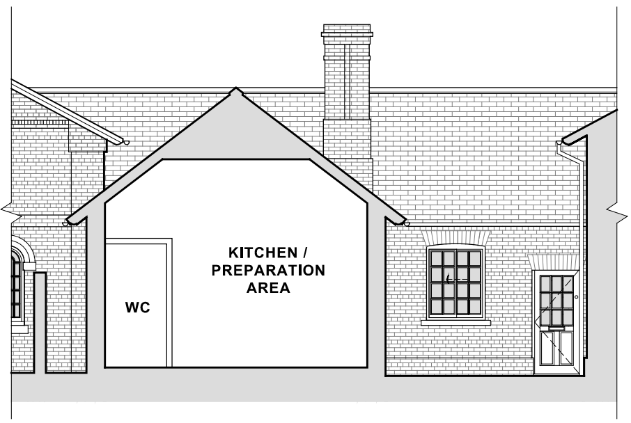
EXISTING SECTION C-C 1:100 @ A3
