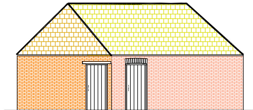
SW ELEVATION
