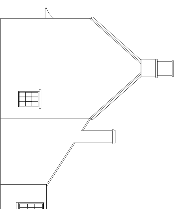
Right Elevation
