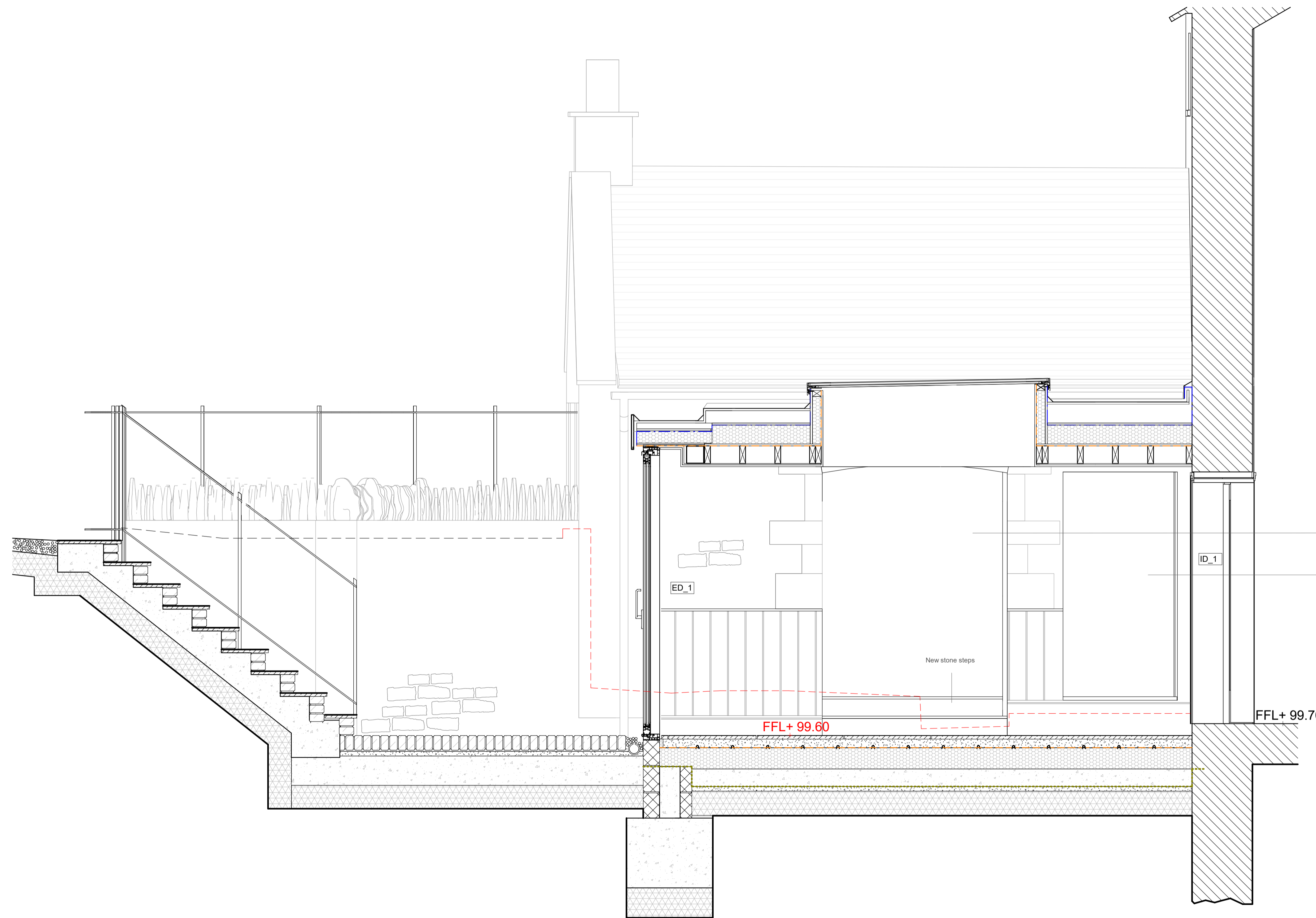
Propsoed - Section AA 1 : 20
