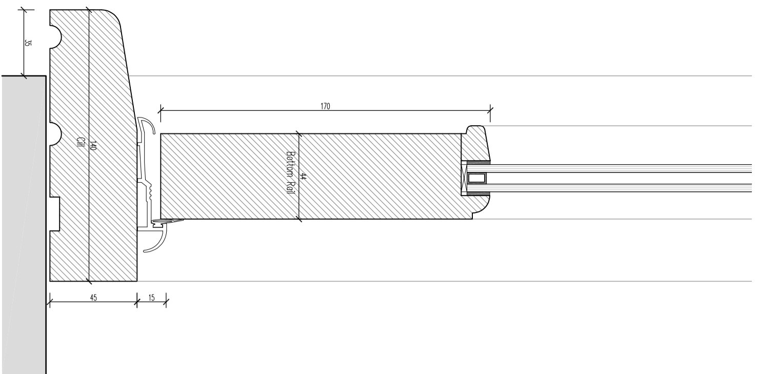
Vertical Door Section 1:2
