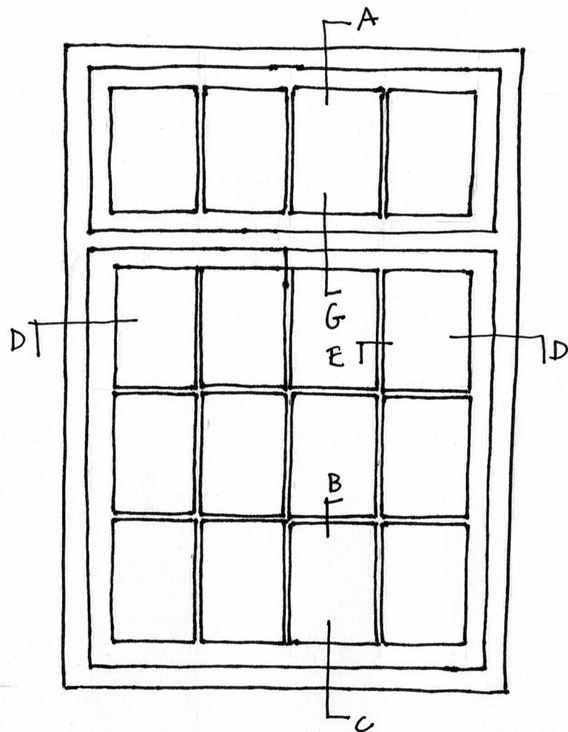
W14 1:10.
