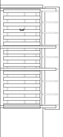
ELEVATION 2
