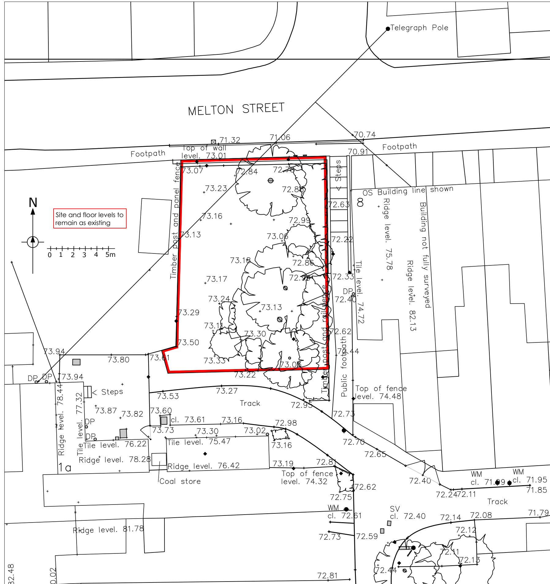
Site plan 1:200
